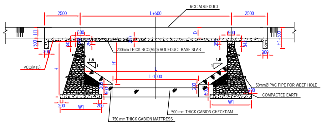
LONGITUDINAL SECTION AT A-A
